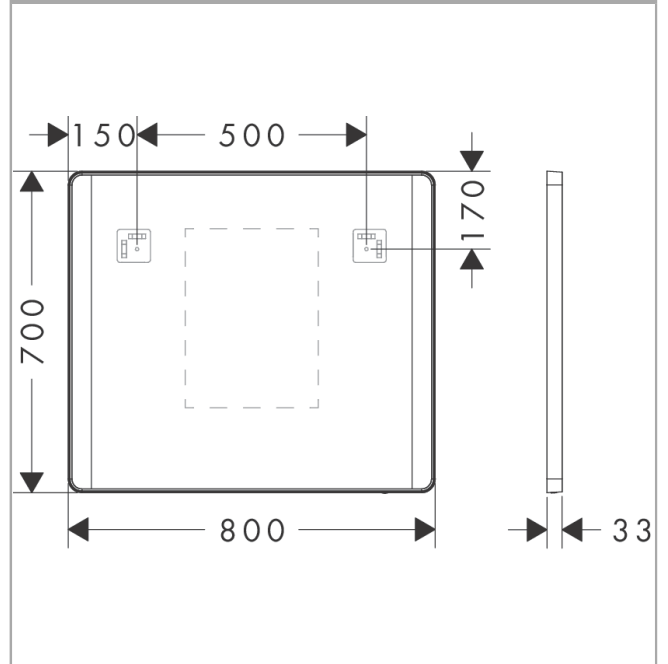
Maattekening
