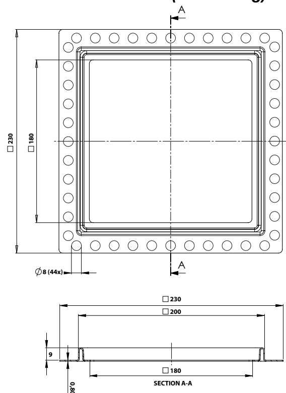
RP20 200x200 mm (9 mm hoog)
