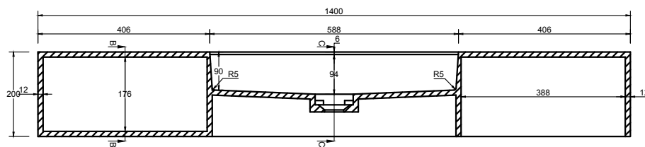
SECTION A-A
