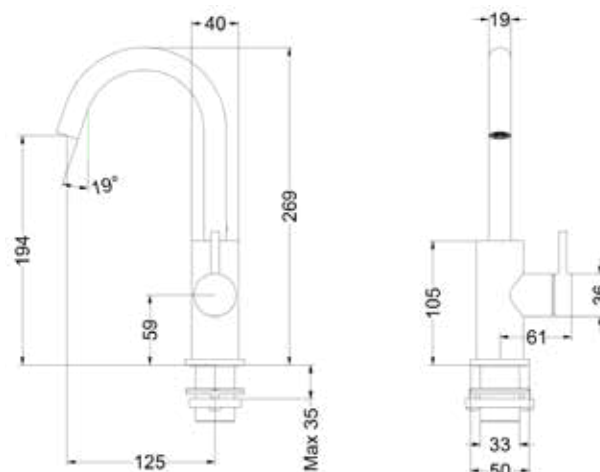
Bond eenhendel wastafelmengkraan, opbouw, met draaibare uitloop
