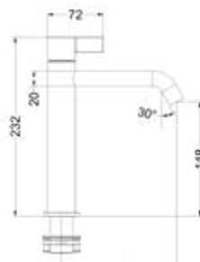
Pact eenhendel wastafelmengkraan, opbouw, model M
