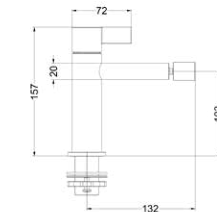
Pact eenhendel bidetmengkraan, opbouw
