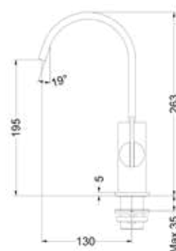
Pact eenhendel wastafelmengkraan, opbouw, met draaibare cascade uitloop
