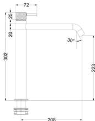
Nexus eenhendel wastafelmengkraan, opbouw, model L
