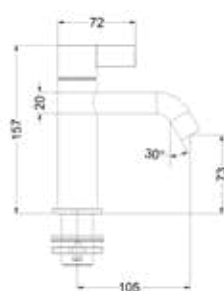
Pact eenhendel wastafelmengkraan, opbouw, model S
