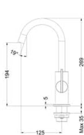
Pact eenhendel wastafelmengkraan, opbouw, met draaibare uitloop
