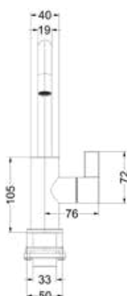
Pact eenhendel wastafelmengkraan, opbouw, met draaibare uitloop
