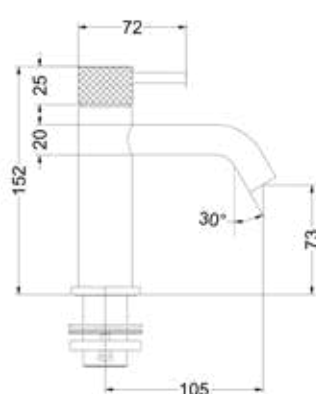
Nexus eenhendel wastafelmengkraan, opbouw, model S
