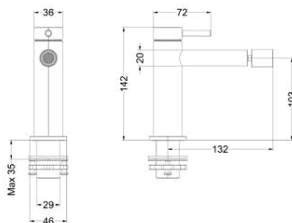
Bond eenhendel bidetmengkraan, opbouw
