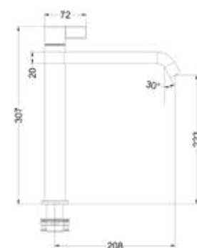
Pact eenhendel wastafelmengkraan, opbouw, model L
