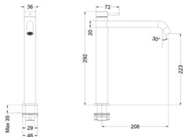
Bond eenhendel wastafelmengkraan, opbouw, model L
