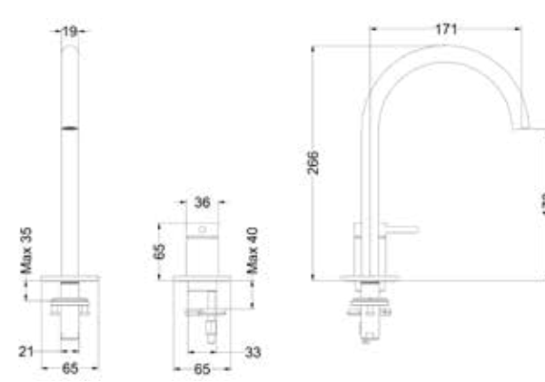
Bond eenhendel wastafelmengkraan, opbouw, 2-gats bladmontage met uitloop
