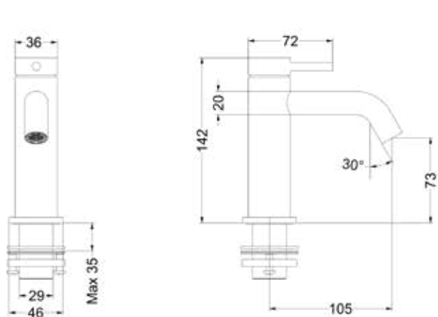
Bond eenhendel wastafelmengkraan, opbouw, model S
