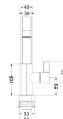
Pact eenhendel wastafelmengkraan, opbouw, met draaibare cascade uitloop
