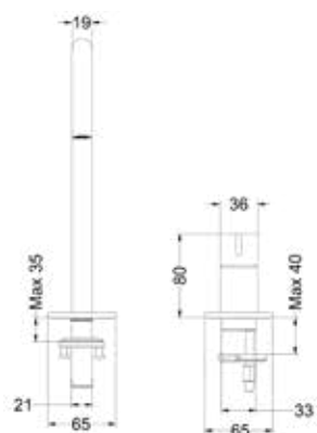
Pact eenhendel wastafelmengkraan, opbouw, 2-gats bladmontage met uitloop
