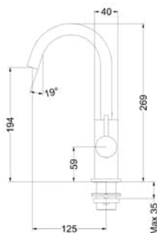
Nexus eenhendel wastafelmengkraan, opbouw, met draaibare uitloop
