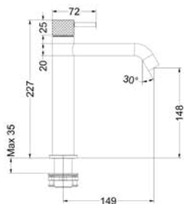
Nexus eenhendel wastafelmengkraan, opbouw, model M
