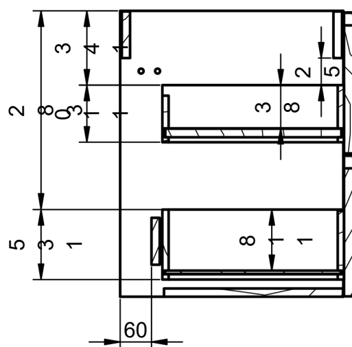
B-B ( 1 : 10 )
