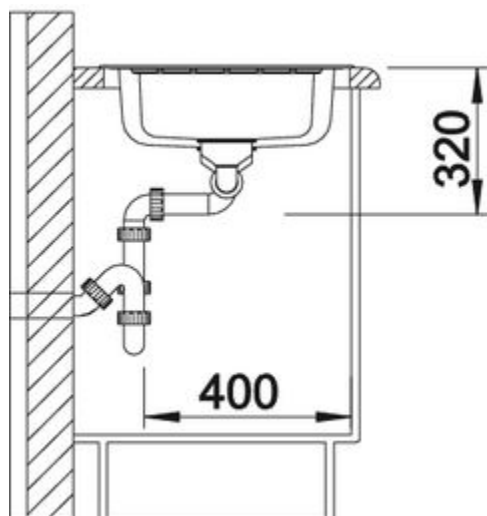
Zijaanzicht
