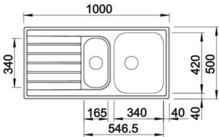
Bovenaanzicht
