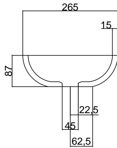
A-A SECTION
