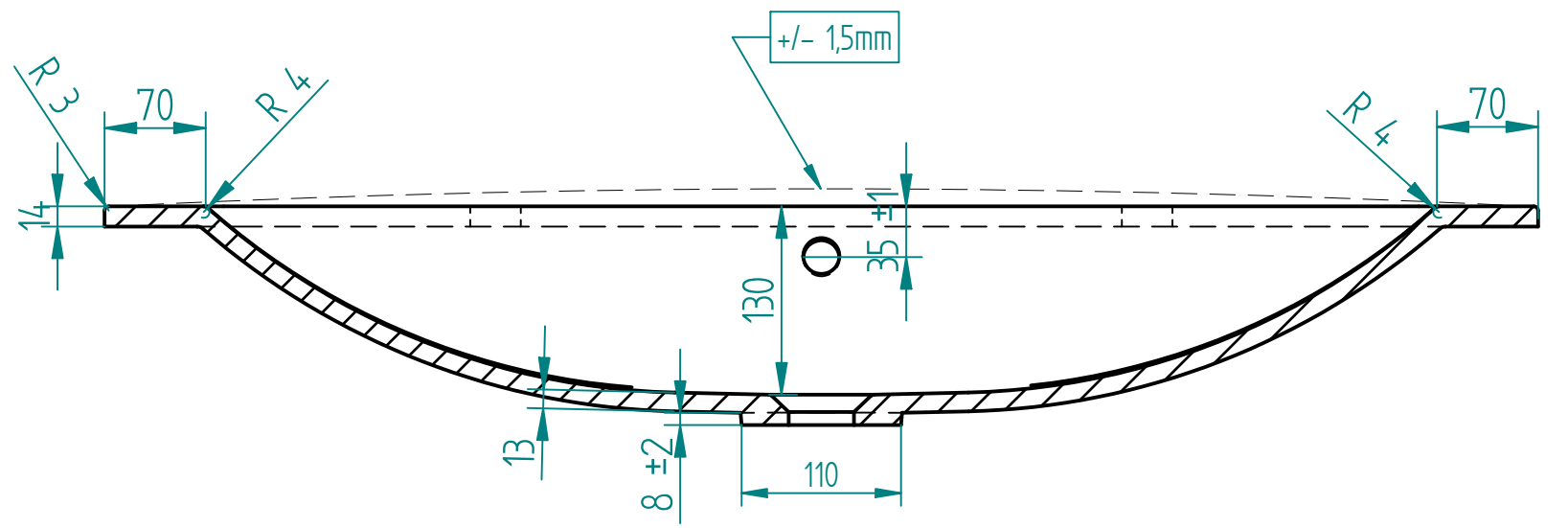
SECTION A-A
