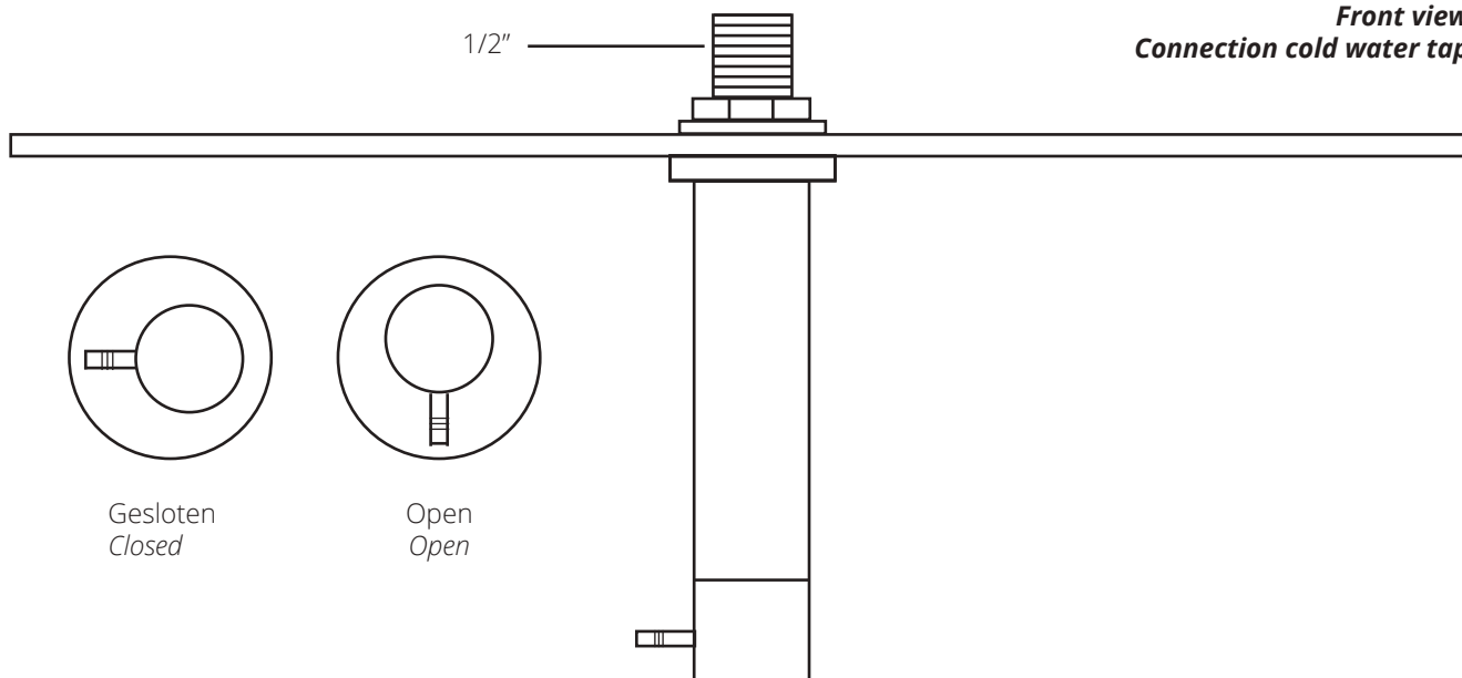
Zijaanzicht koudwaterkraan-aansluiting Side view Connection cold water tap
