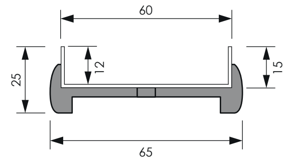
Zijaanzicht met afstandhouder
