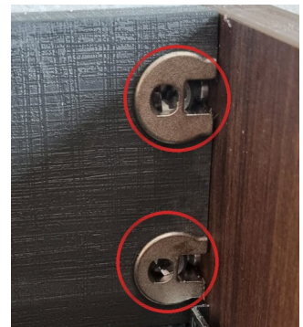
The round connectors (circled in red) De ronde verbinders (rood omcirkeld) Les raccords ronds (entourés en rouge)
