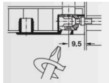
Screwdriver at an angle (approx. 25°) in the connector Schroevendraaier schuin (ca. 25°) in de verbinder Tournevis incliné (env. 25°) dans le raccord
