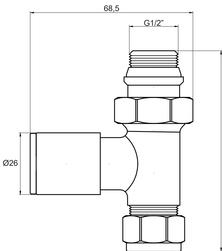
Radiatorkraan
