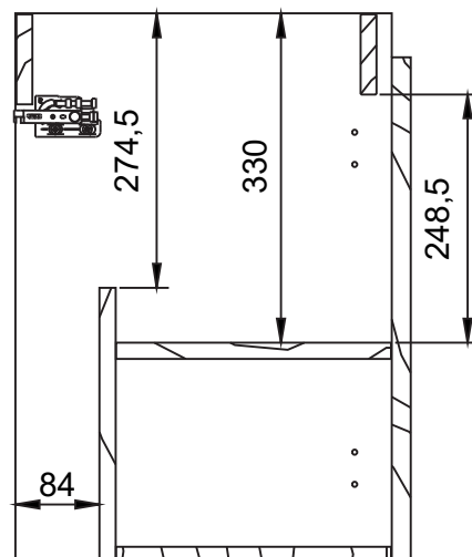
B-B ( 1 : 8 )
