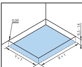
Voorbereiding montage
