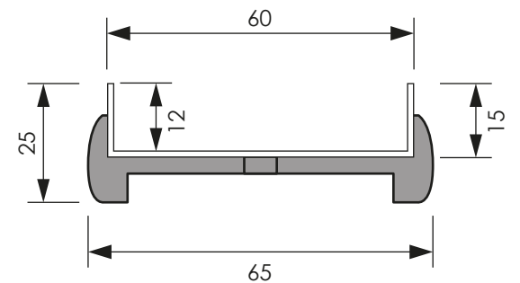
Zijaanzicht met afstandhouder
