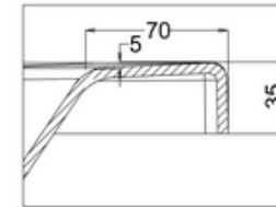
D SCALE 1:2
