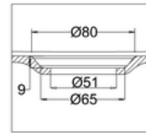
C SCALE 1:2
