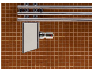
Aansluitblok kap kort voor cv gebruik
