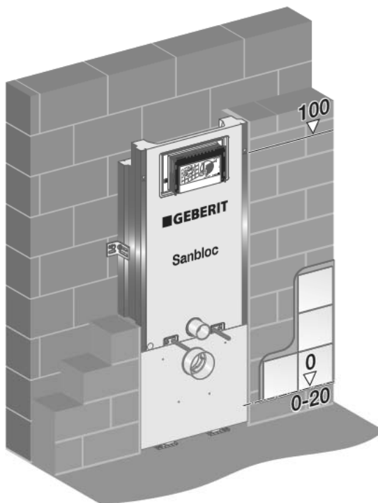
Vóór een muur en vervolgens ommetseld
