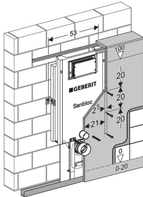
6 a. Voorbeeld van een Sanbloc wc-element in een lichte voorzetwand
