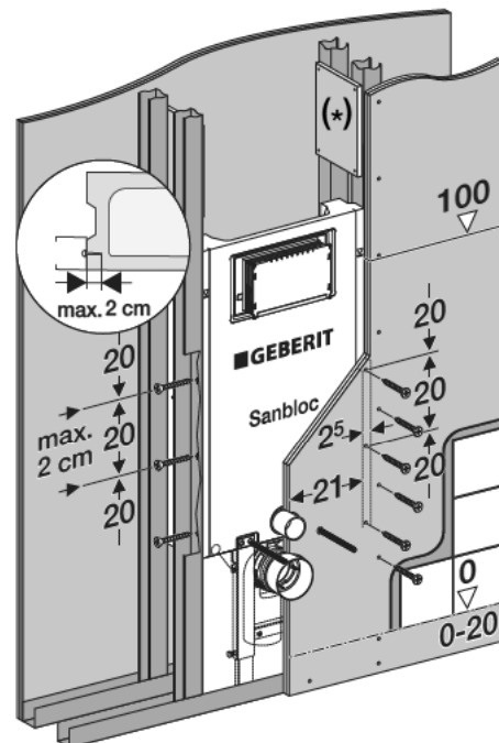
6 b. Voorbeeld van een Sanbloc wc-element in een lichte scheidingswand
