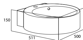
5998 Wasbak (excl. kraan en waste) Lavabo (robinet et vidange non compris)
