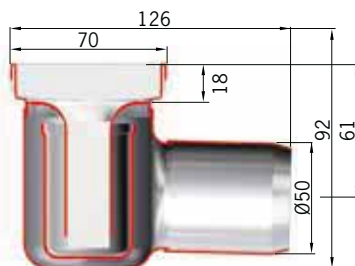
Standaard versie met 50 mm stankslot
