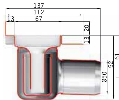
Standaard versie met muurflens en 50 mm stankslot
