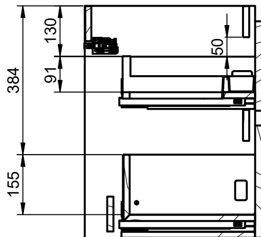
A-A ( 1 : 10 )
