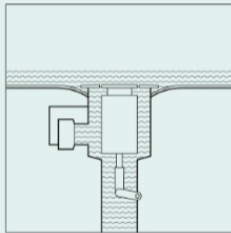
BADAFVOER GESLOTEN, OVERLOOP OPEN
