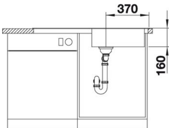
Vooraanzicht
