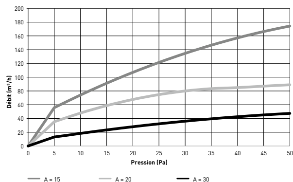
Courbe de pression / débit DucoVent Basic
