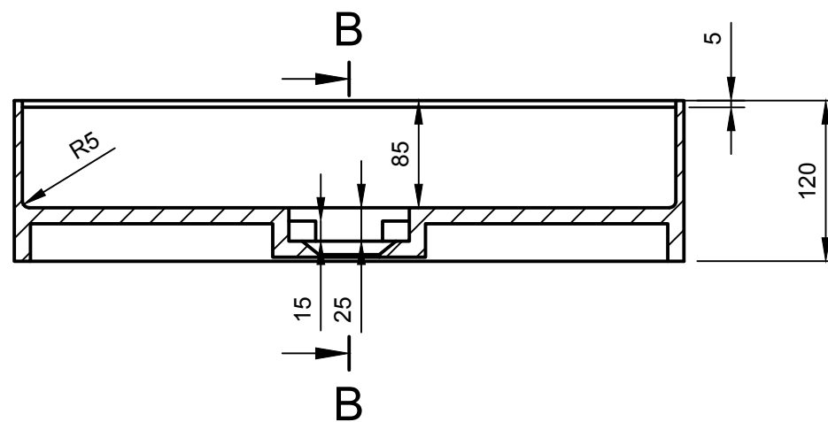
A-A (1:5)
