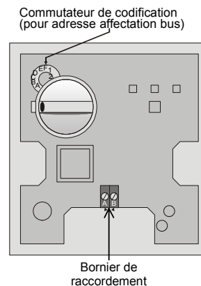
Fig. 2. Vue interne du boîtier SDW 10 (capot enlevé)
