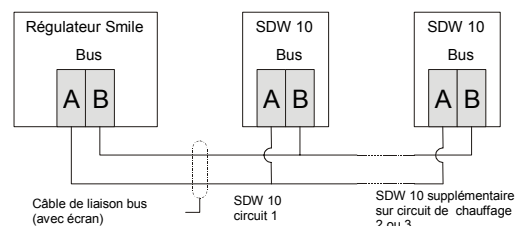
Fig. 3. Raccordement électrique au régulateur
