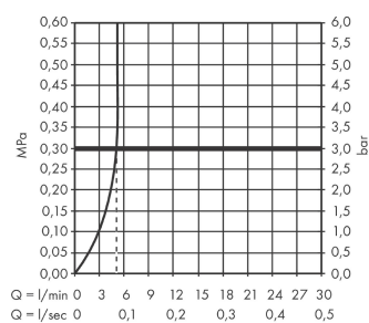
Doorstroomdiagram
