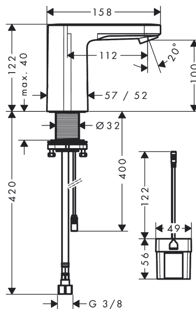
Maattekening
