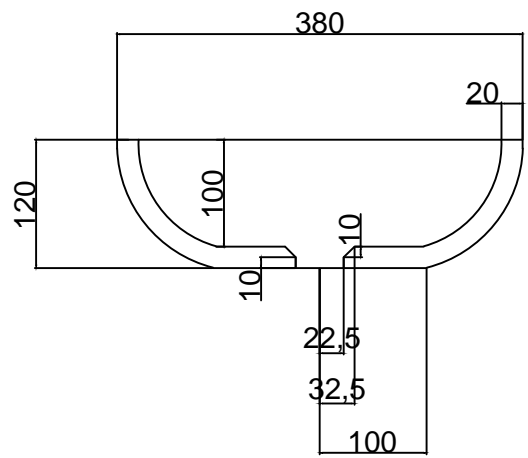
A-A SECTION
