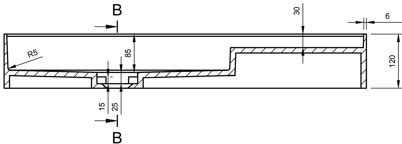
A-A (1:5)
