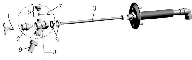
Producttekening
