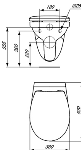
Wandcloset diepspoel 520 mm exclusief closetzitting
