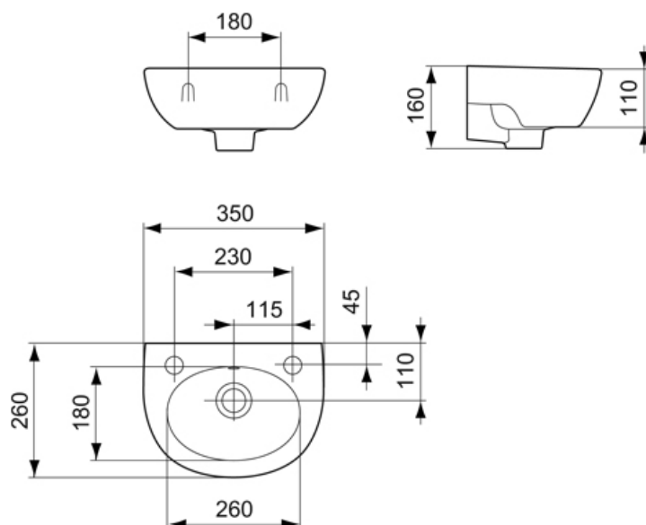
Fontein 350 x 260 mm met kraangat rechts met overloop
