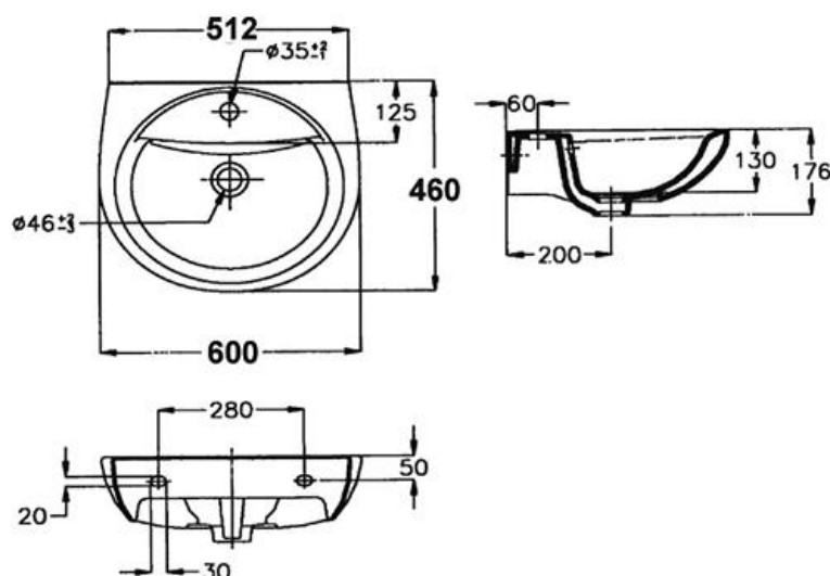
Wastafel 600 mm met kraangat met overloop
