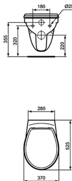
Wandcloset spoelrandloos exclusief closetzitting
