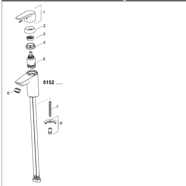
Producttekening
