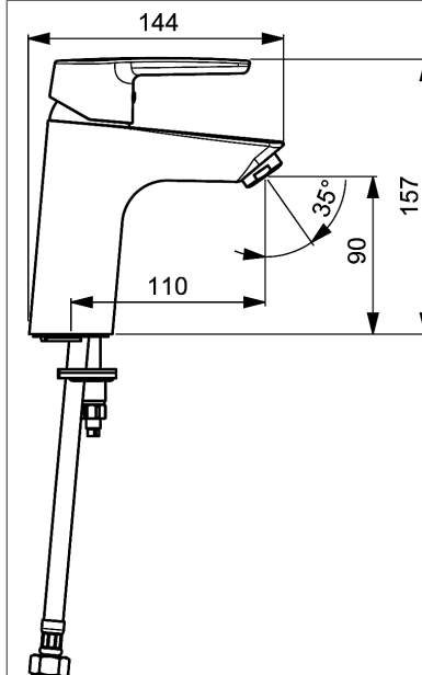
Producttekening
