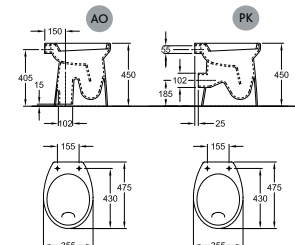
Staand Closet I Cuvette à poser Standing closet-pan +6 cm 35,5 x 47,5 cm
