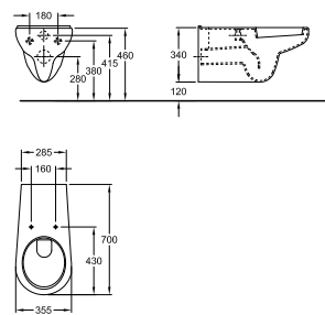
Wandcloset verlengd I Cuvette suspendue allongée I Extended wallhung closet-pan 35,5 x 70 cm
