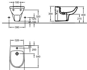
Wandbidet I Bidet suspendu Wallhung bidet 35,6 x 54 cm
