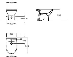
Staand bidet I Bidet à poser Standing bidet 35,6 x 54 cm
