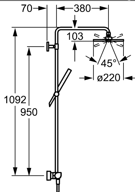
Producttekening
