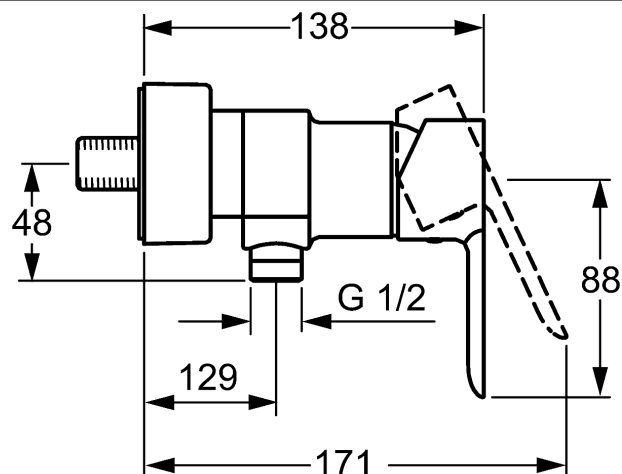
Producttekening
