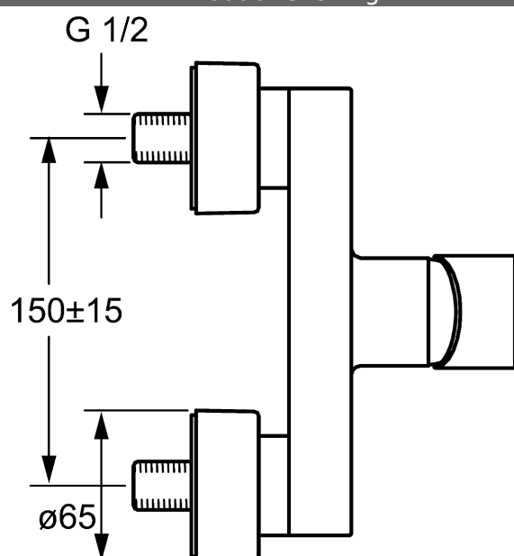
Producttekening
